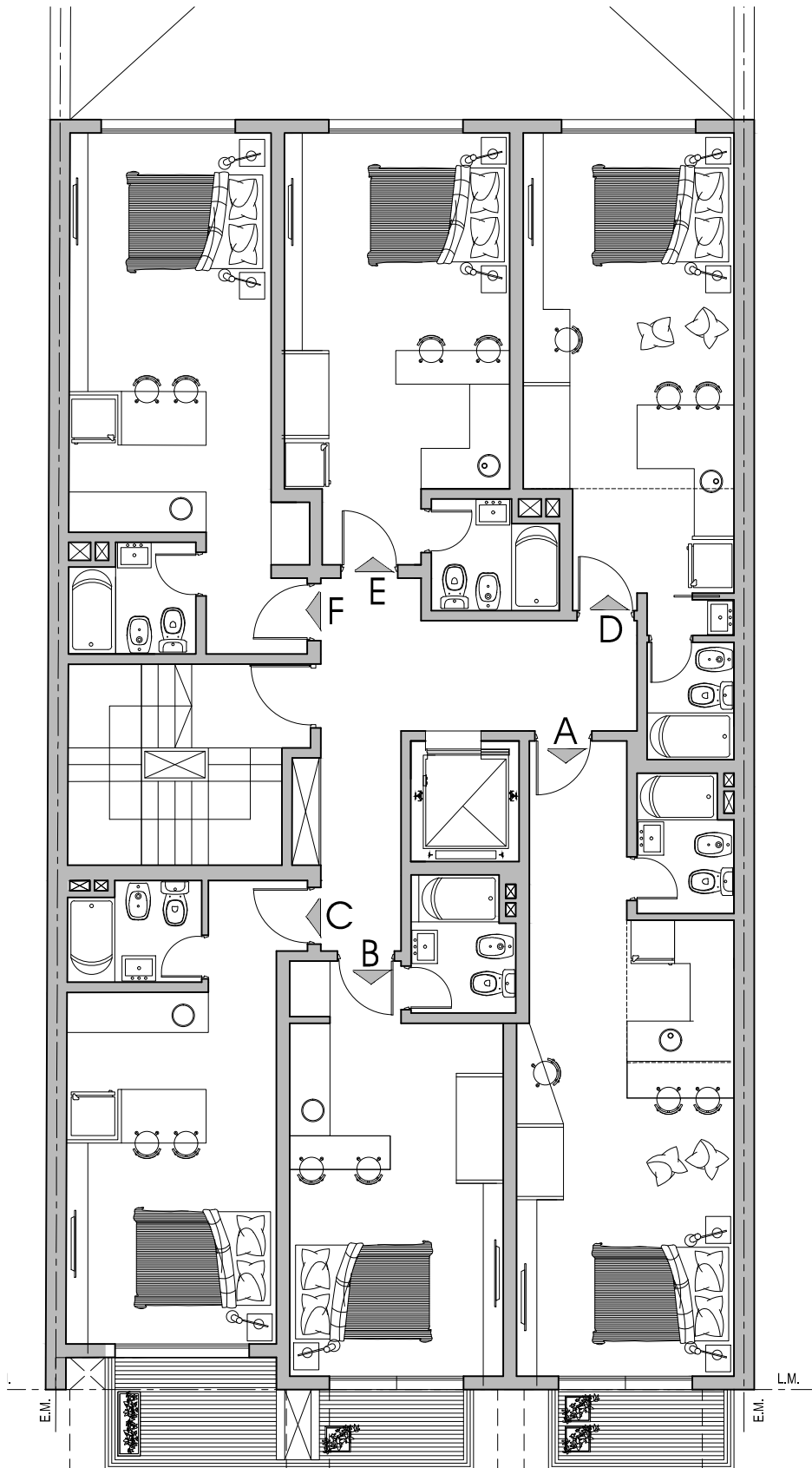
PLANTA DE UBICACION
